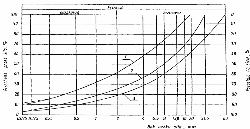
Rysunek 1. Pole dobrego uziarnienia kruszywa przeznaczonych na podbudowy
